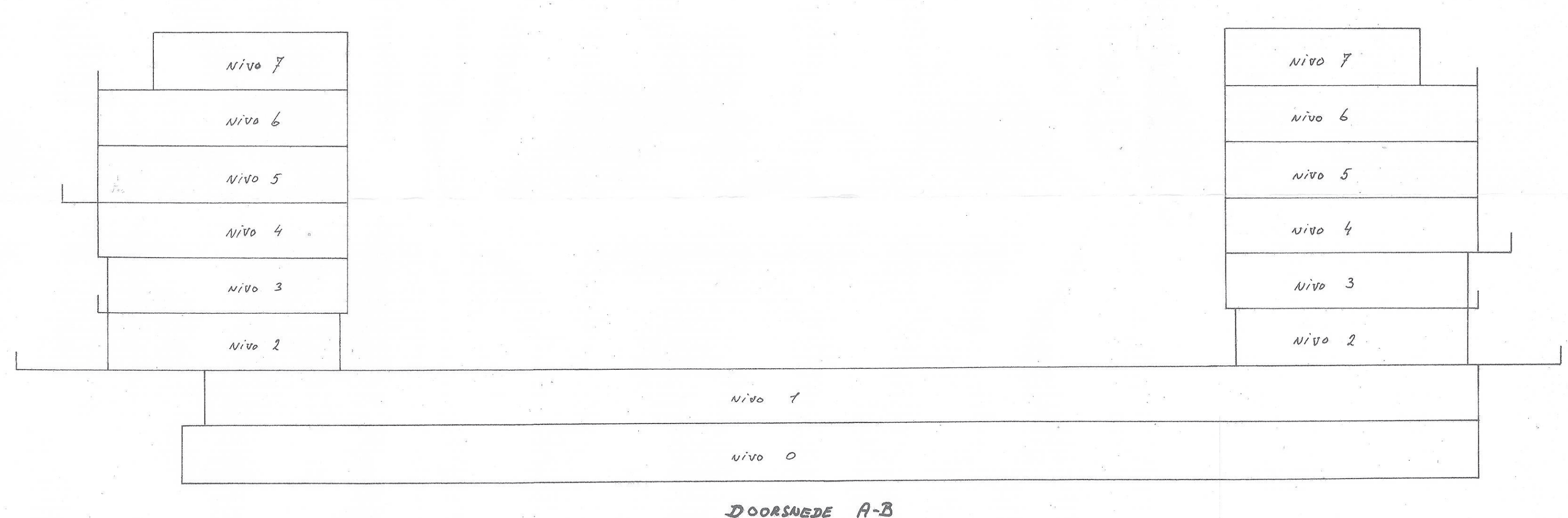
Doorsnede A-B 1:200
