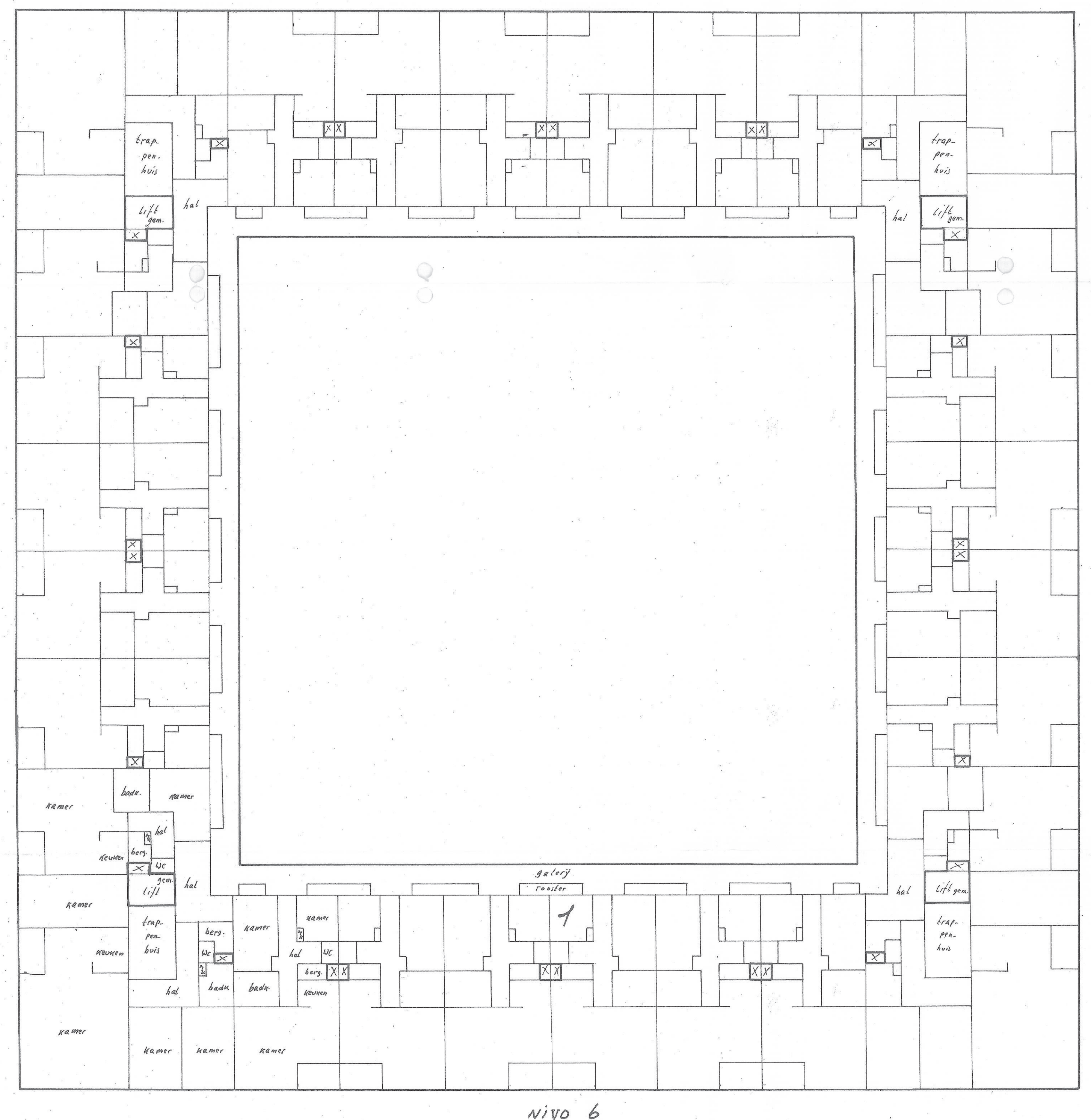
Nivo 6 1:200
