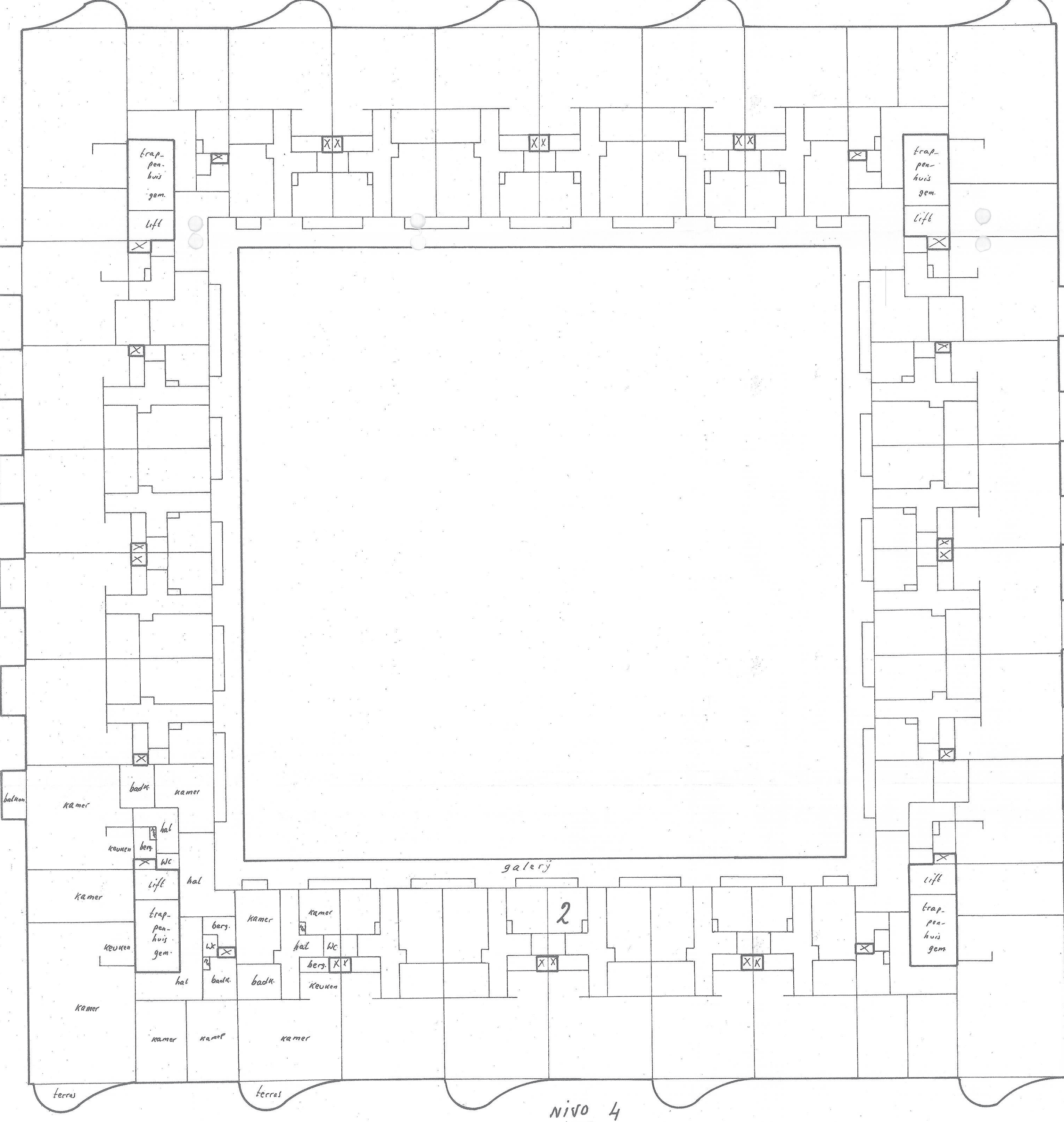
Nivo 4 1:200
