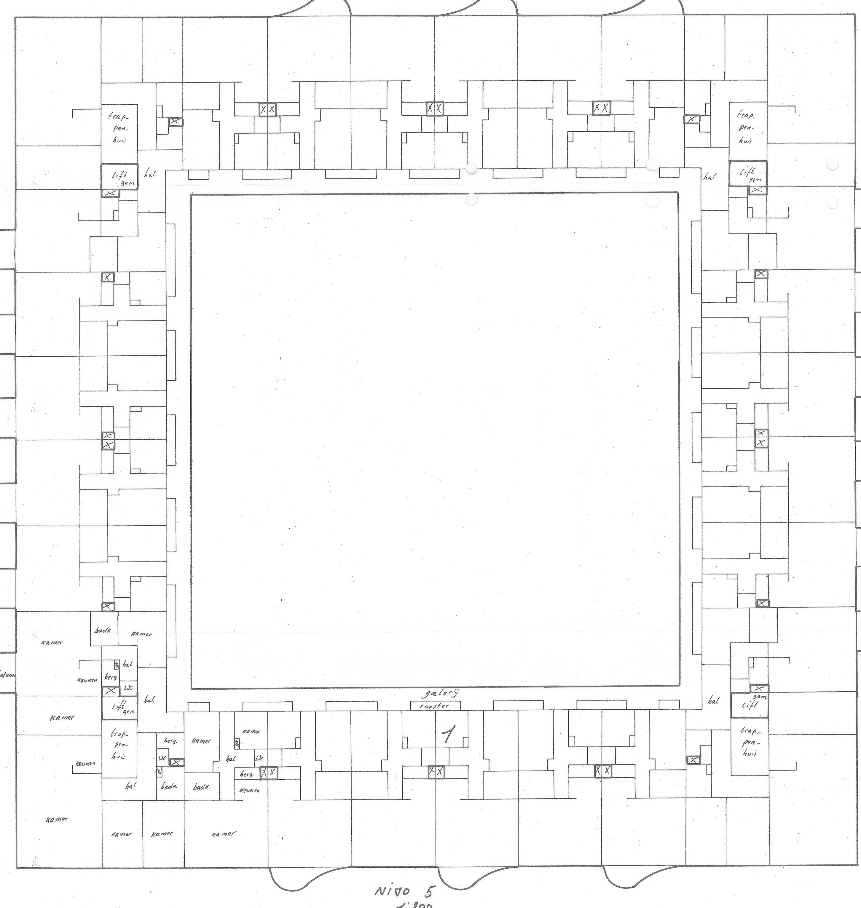
Nivo 5 1:200
