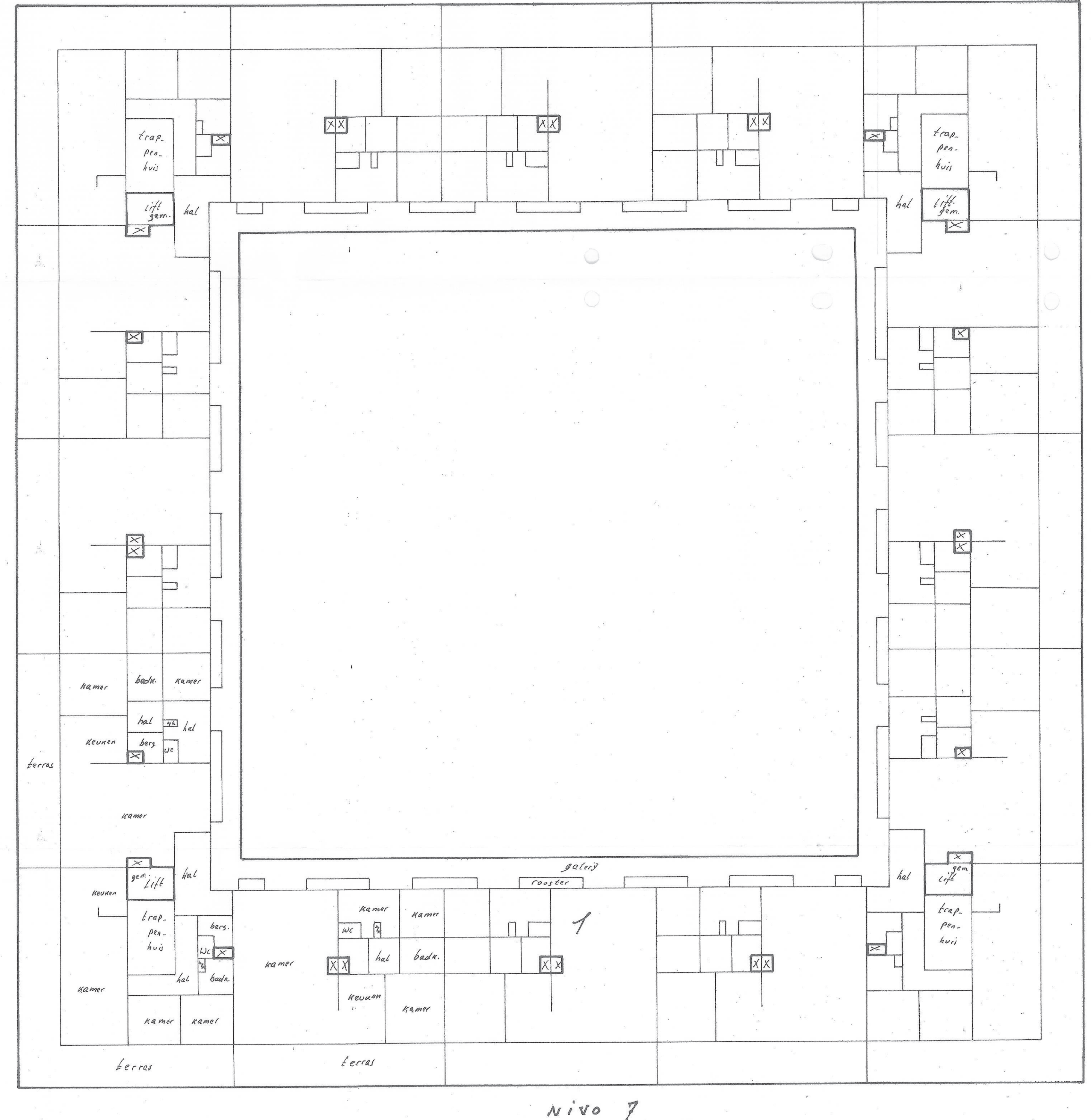
Nivo 7 1:200
